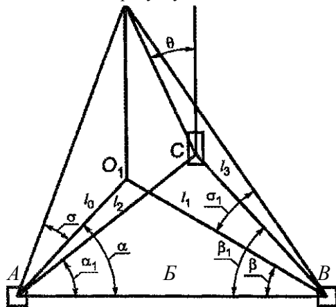
А и В — пункты оптических измерителей; С — пусковая установка; О — точка срабатывания ПИ; О 1 — проекция точки срабатывания ПИ на горизонтальную плоскость
